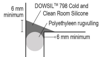
Figuur 3: Driehoeksvoeg.
